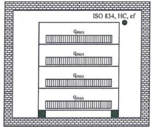
Fig. 2: SEZIONE VERTICALE
