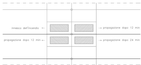
Scenario S3
